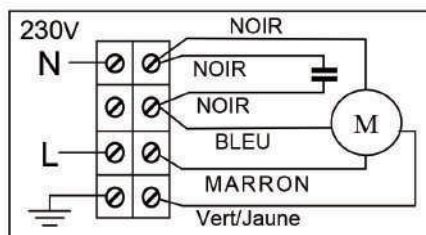
Schéma de câblage Monophasé 230VAC
