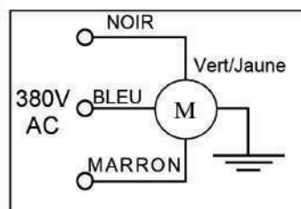
Schéma Triphasé 380VAC
